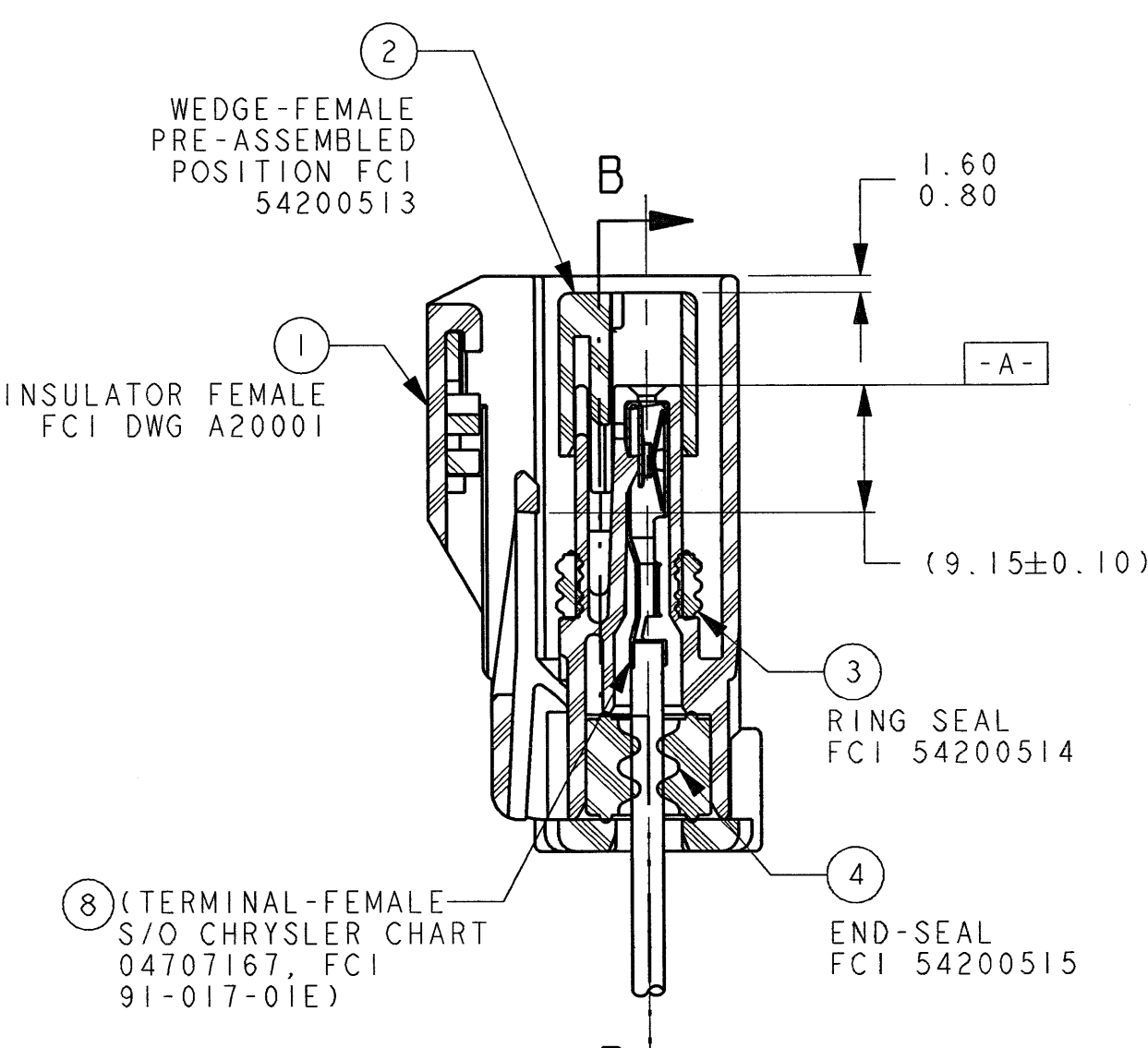
SECTION A-A
